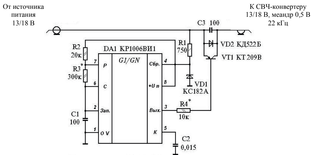
Рис. 4. Схема формирователя тонального сигнала 22 кГц
