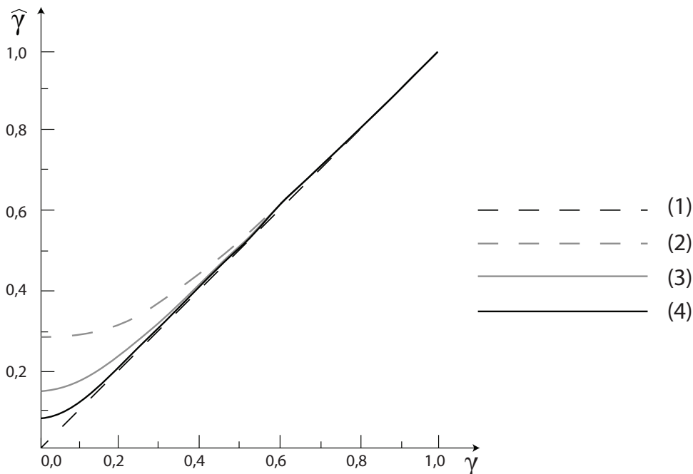
Рис. 2. Зависимость оценки величины когерентности \hat{\gamma} от ее истинного значения. Линия (1) соответствует теоретической зависимости, линия (2) — размеру области усреднения 3 \times 3 , линия (3) — размеру области усреднения 7 \times 7 , линия (4) — размеру области усреднения 15 \times 15
