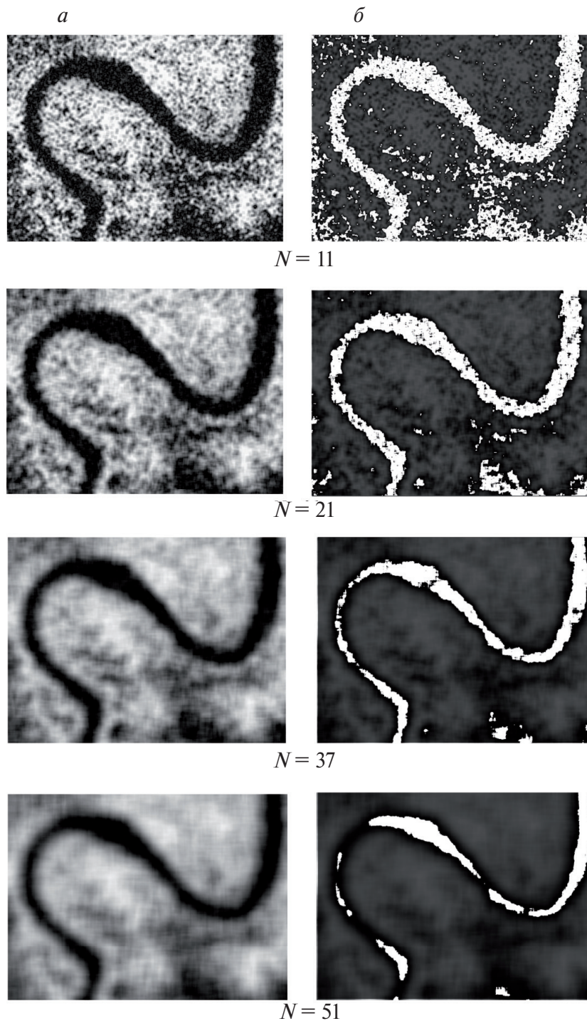
Рис. 5. Моделирование карт когерентности PCA-пары при различных размерах области усреднения:
