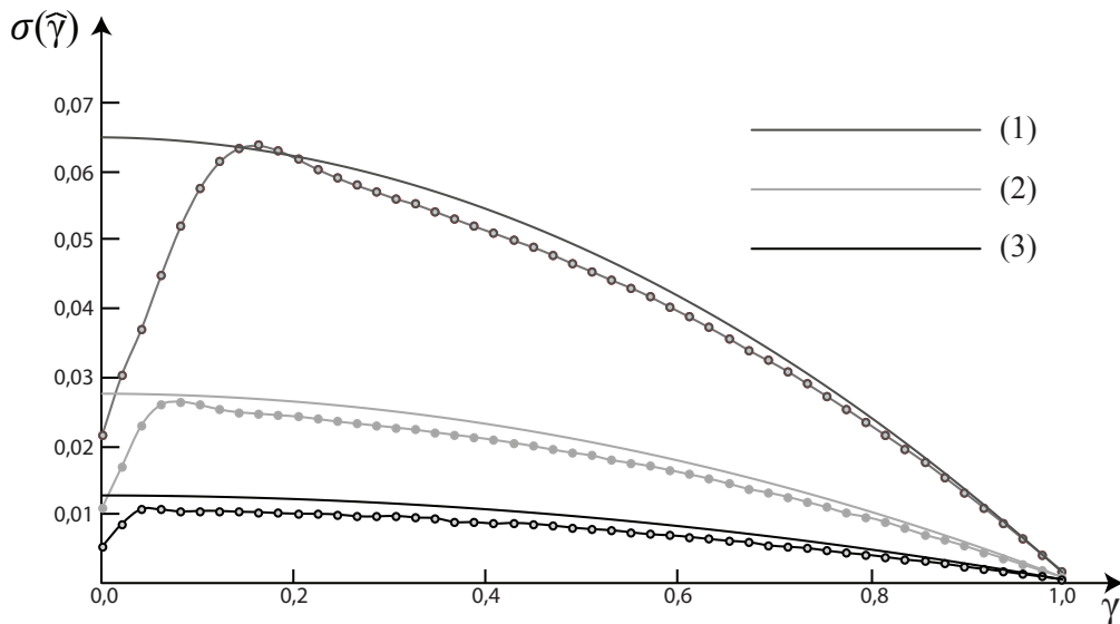
Рис. 4. Зависимость СКО оценки когерентности \sigma_{\hat{\gamma}} от ее истинного значения. Линия (1) соответствует размеру области усреднения 11 \times 11 , линия (2) — размеру области усреднения 37 \times 37 , линия (3) — размеру области усреднения 51 \times 51 . Пунктирной линией показана теоретическая зависимость
