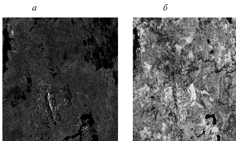
Рис. 6. Одно из двух изображений РСА-пары, полученное с помощью спутниковой системы ALOS PALSAR — а; карта когерентности, построенная по приведенным данным (размер области усреднения составляет 21 \times 21 ) — б
