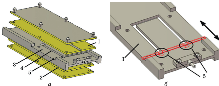
Рис. 1. Модель МПЩ-перехода с П-образным щелевым резонатором переменной длины
