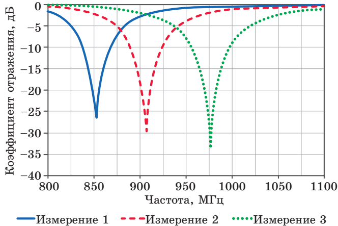
Рис. 6. Зависимость коэффициента отражения ( S_{11} ) МПЩ-перехода в диапазоне частот от положения перемычки при заполнении щелевого резонатора диэлектриком Fig. 6. The reflection coefficient ( S_{11} ) in the frequency range vs. the position of the bridge with dielectric material filling of the slot resonator
