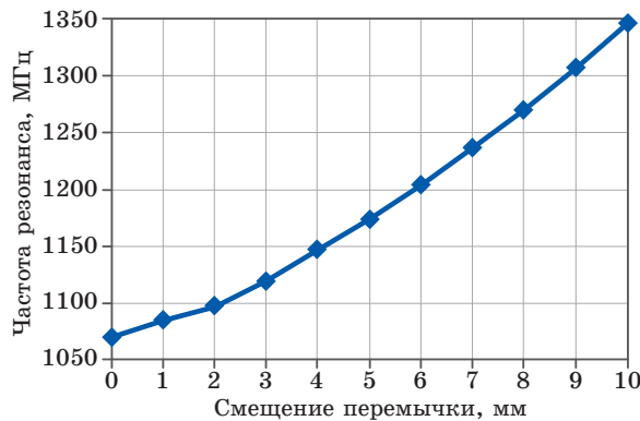
Рис. 4. Зависимость частоты резонанса МПЩ-перехода с П-образным щелевым резонатором от смещения перемычки
